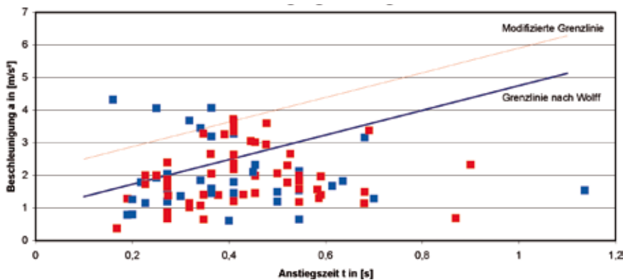
BILD 6: Beschleunigungen und Anstiegszeiten bei den eigenen Versuchen und den Versuchen von Wolff sowie die jeweiligen Grenznlinien
