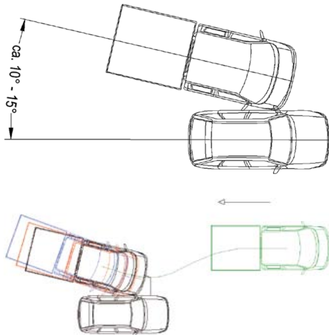
BILD 4: Anstoßwinkel beim Kollisionsversuch 2
